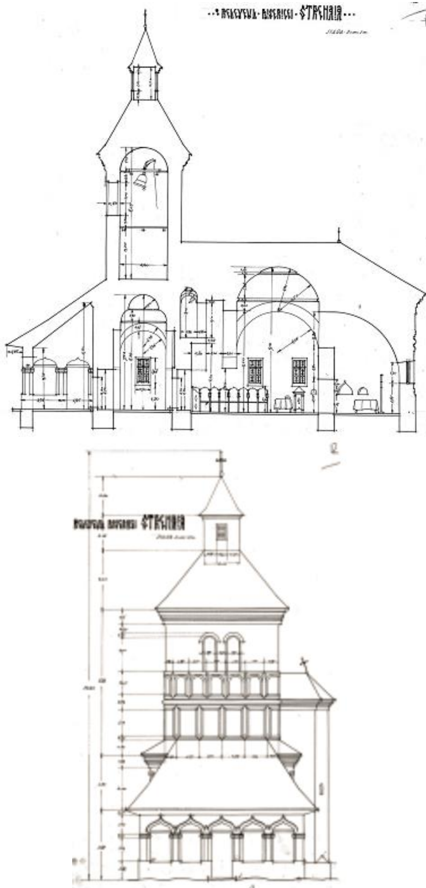
80. Biserica Sfânta Treime a Mănăstirii din Strehaia, ctitorită de Matei Basarab (secțiunea longitudinală și fațada vestică)
