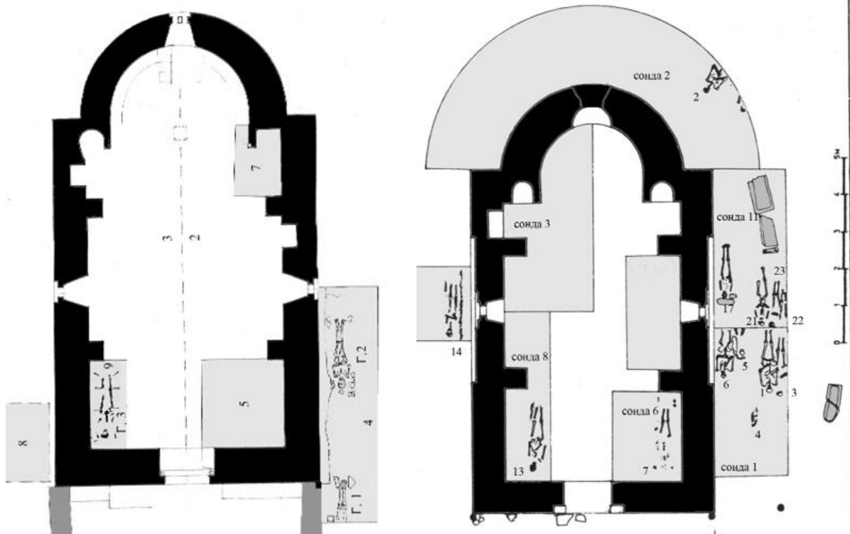
11. Planurile Bisericilor Sân Nicoară de la Curtea de Argeș, Sfântul Nicolae de la Șumnik și Sfântul Nicolae (ulterior Sfânta Parascheva ) de la Radoșić
