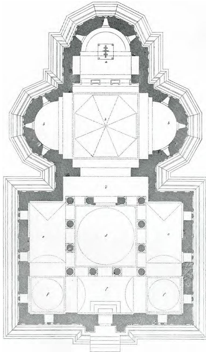
83. Planul Bisericii Sfintei Marii rezidite din temelii de Neagoe Basarab la Argeș (1517)
