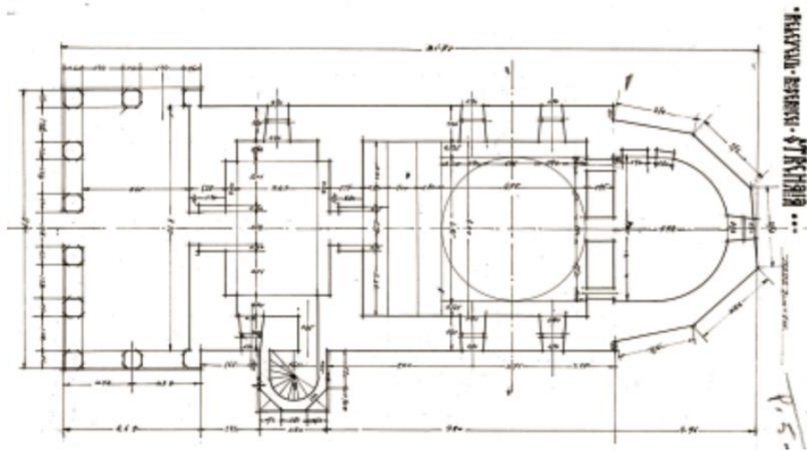
80. Biserica Sfânta Treime a Mănăstirii din Strehăia, ctitorită de Matei Basarab (planul bisericii)
